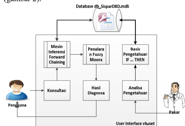
Gambar 2. Arsitektur Sistem Pakar
