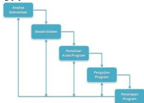
Gambar 1. Diagram langkah-langkah metode waterfall
