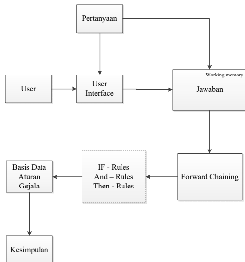
Gambar 3. Mesin Inferensi
