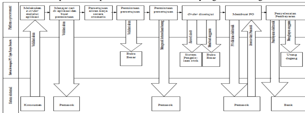
Gambar 3. Blueprint Arsitektur Sistem Informasi e-Procurement
