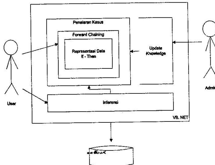
Gambar 3. Model Arsitektur Perancangan Sistem Pakar Diagnosa Penyakit Ikan Komet
