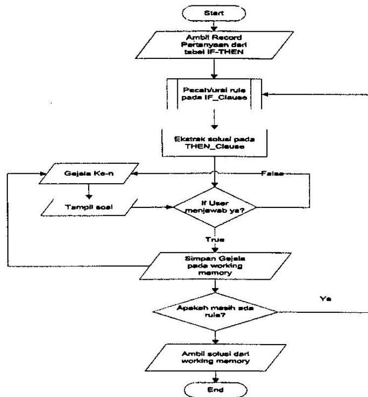
Gambar 6. Mekanisme Inferensi Sistem Pakar Diagnosa Penyakit Ikan Komet
