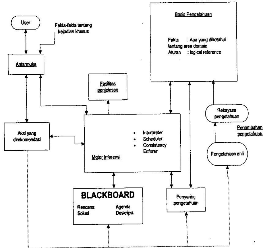
Gambar 2. Strukur Komponen Sistem Pakar
